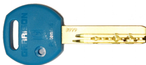
Jamkový jednoradový kľúč
